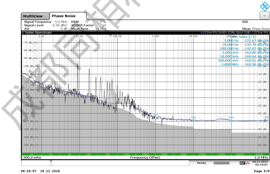
5MHz 相位噪声测试图
