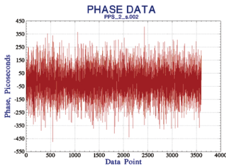
上图为节点时间同步测试数据
