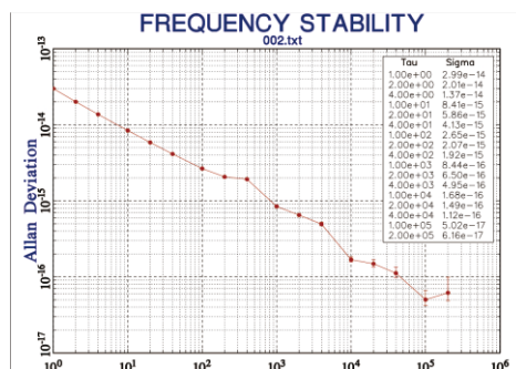
上图为节点频率附加稳定度测试数据
